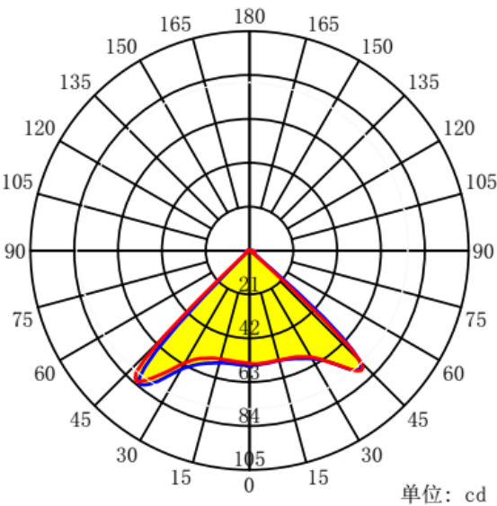
配光曲线
